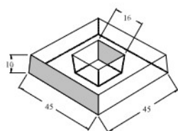
Tête carrée
