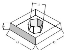
Tête hexagonale
